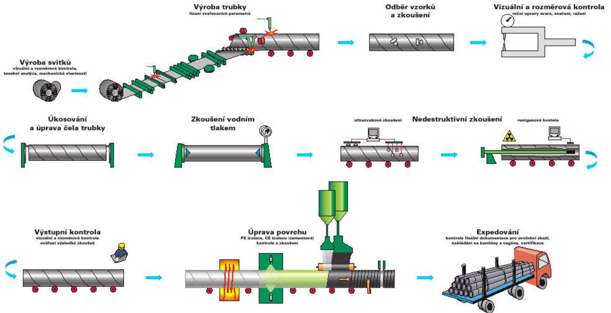
Technologický tok výroby trubek se šroubovicovým svarem v NH Vítkovice
