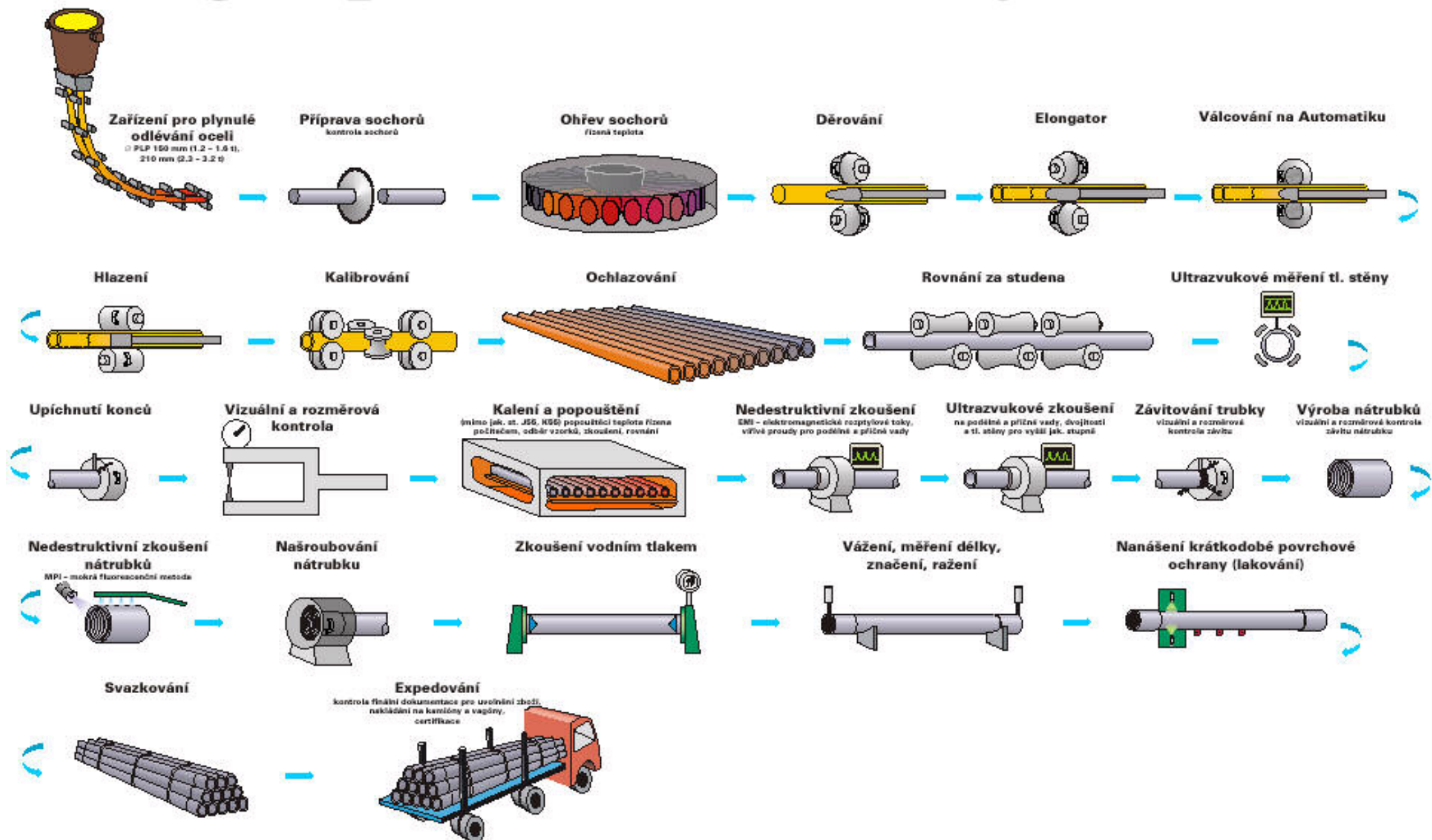
Technologický tok výroby pažnicových trubek v NH Vítkovice
