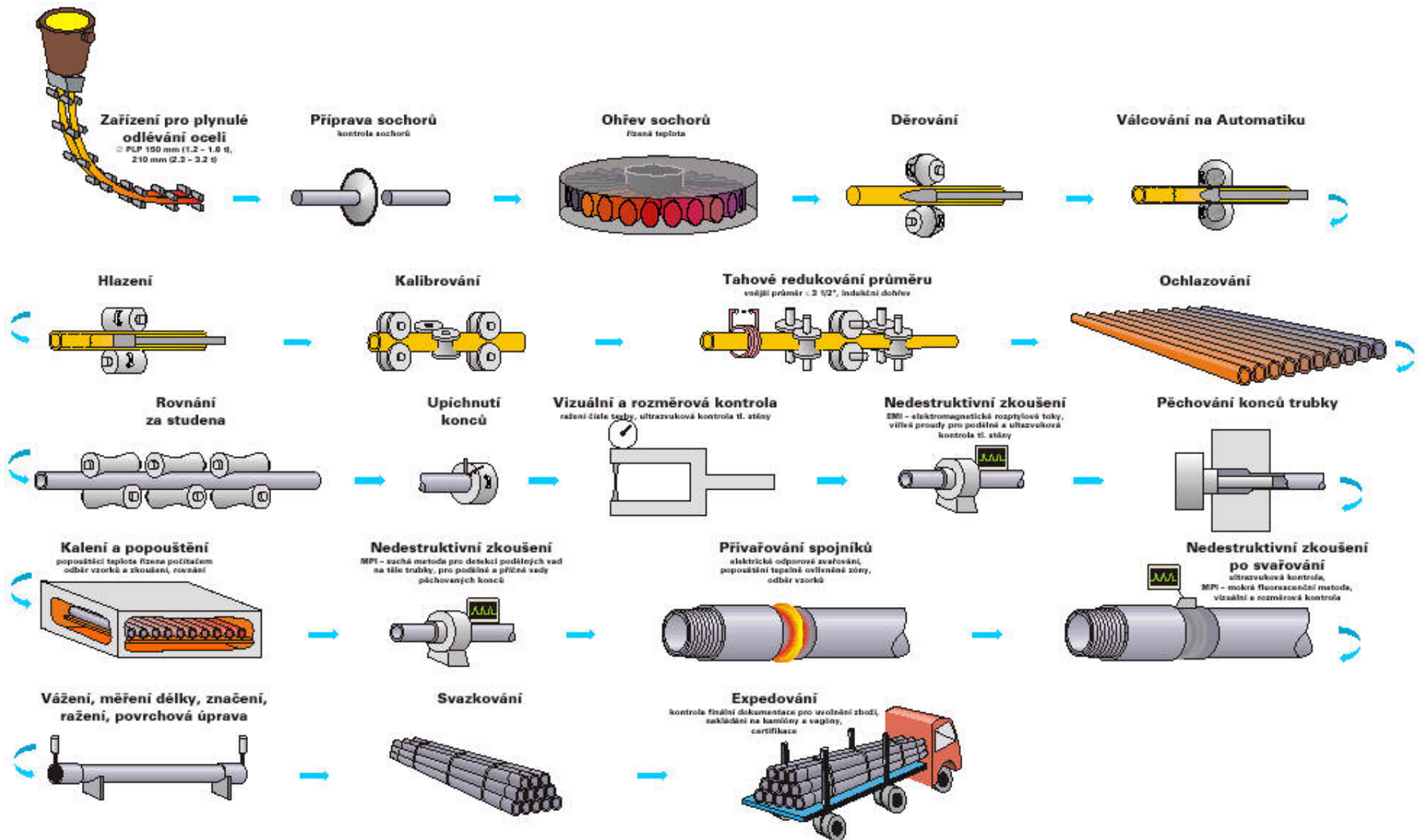
Technologický tok výroby vrtných trubek v NH Vítkovice
