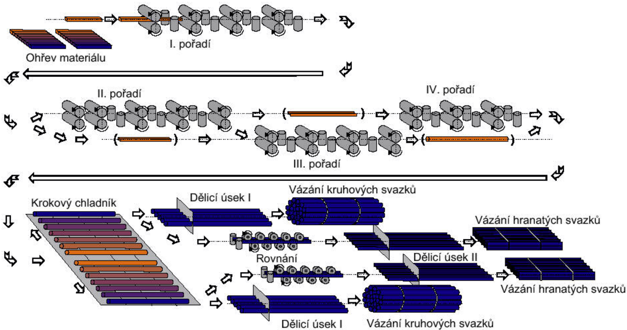
Středojemná trať v NH Vítkovice
