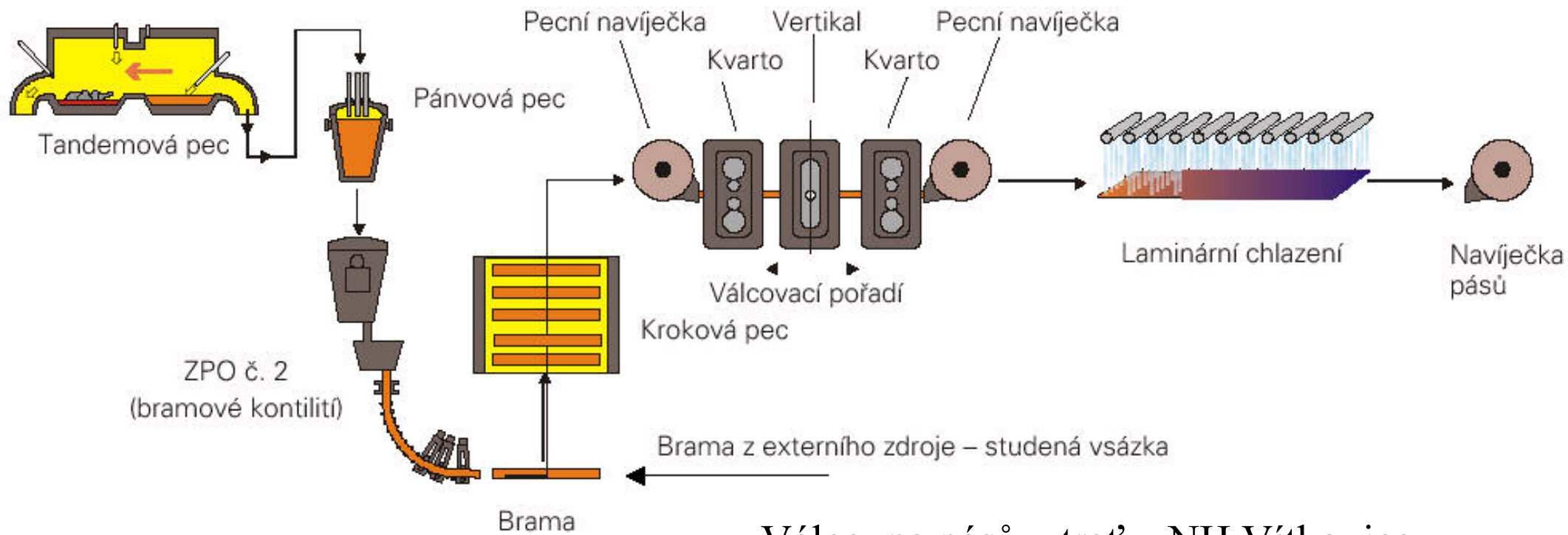
Válcovna pásů – trať v NH Vítkovice
