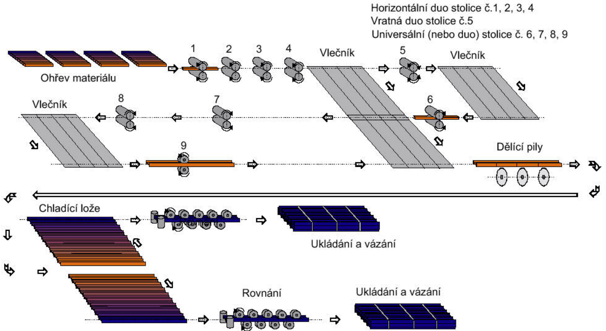
Hrubá profilová trať HCC v NH Vítkovice
