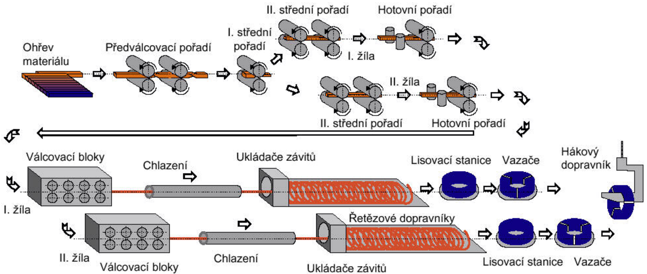
Kontidráťová trať v NH Vítkovice
