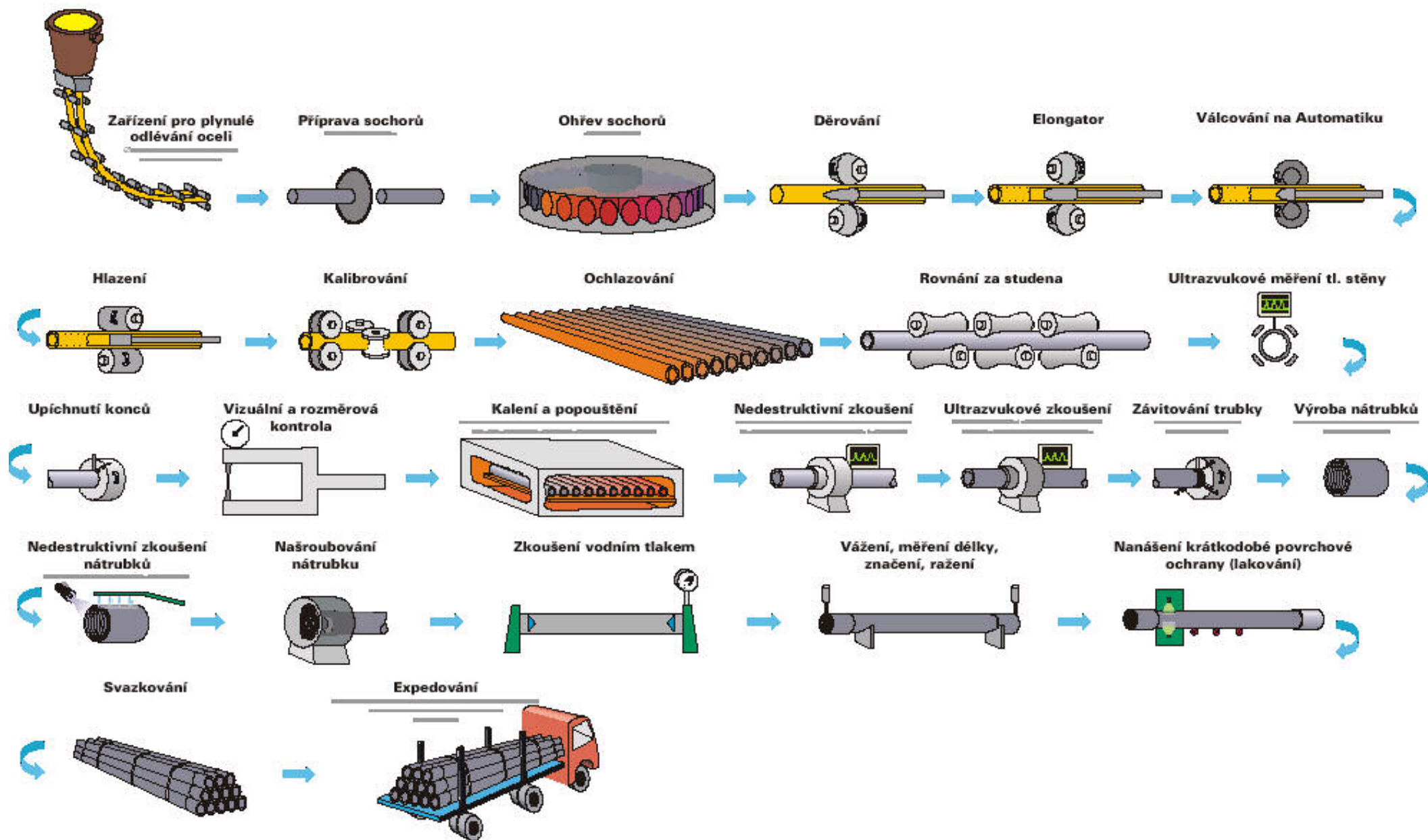
Technologický tok výroby bezešvých trubek v NH Vítkovice
